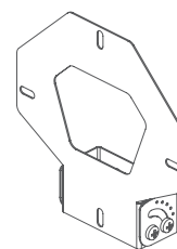
Uchwyt montażu kątownego / 0° - 90° mounting support
